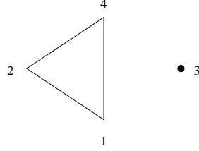
Figura 2: un complejo simplicial
