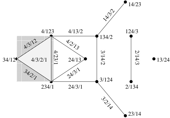
Figura 5: un complejo de extensiones lineales
