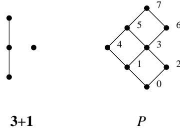
Figura 7: el poset \mathbf{3} + \mathbf{1} y otro poset que no es libre de \mathbf{3} + \mathbf{1}
