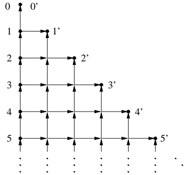
Figura 6: el grafo de Gessel y Viennot
