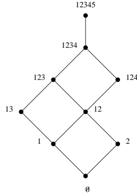
Figura 4: un retículo distributivo
