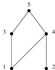
Figura 3: un conjunto parcialmente ordenado
