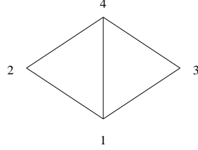
Figura 1: un complejo simplicial
