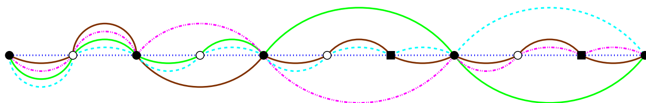
(d) Straighten the new curve to get V_5 .
