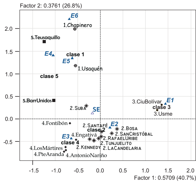
FIGURA 3: Primer plano factorial del ACS de la tabla de contingencia Bogotá. Se destacan las clases mostrando sus centros de gravedad y la clase a la que pertenece cada localidad. Se incluye SE como columna ilustrativa.
