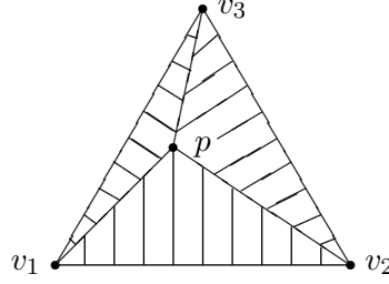
Figure 1. \text{ch}(v_1, v_2, v_3) = \text{ch}(v_1, v_2, p) \cup \text{ch}(v_1, v_3, p) \cup \text{ch}(v_2, v_3, p) .
